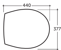
СИДЕНЬЕ С КРЫШКОЙ ГРАНД (ДЮРОПЛАСТ) / СИДЕНЬЕ С КРЫШКОЙ ГРАНД (ДЮРОПЛАСТ С МИКРОЛИФТОМ) GRAND WC SEAT WITH COVER (DUROPLAST) / GRAND WC SEAT WITH COVER (DUROPLAST WITH SOFTCLOSE)
