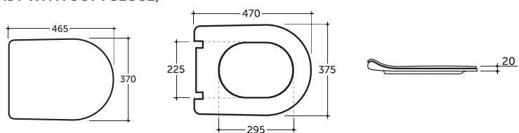
СИДЕНЬЕ С КРЫШКОЙ БЕРГАМО SLIM (ДЮРОПЛАСТ С МИКРОЛИФТОМ) BERGAMO SLIM WC SEAT WITH COVER (DUROPLAST WITH SOFTCLOSE)
