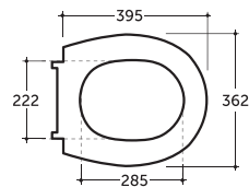
СИДЕНЬЕ С КРЫШКОЙ ГРАНД (ДЮРОПЛАСТ) / СИДЕНЬЕ С КРЫШКОЙ ГРАНД (ДЮРОПЛАСТ С МИКРОЛИФТОМ) GRAND WC SEAT WITH COVER (DUROPLAST) / GRAND WC SEAT WITH COVER (DUROPLAST WITH SOFTCLOSE)
