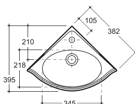
УМЫВАЛЬНИК ВЕРОНА 55 УГЛОВОЙ МЕБЕЛЬНЫЙ SEMI-RECESSED WASH-BASIN VERONA 55 CORNER-MOUNTABLE
