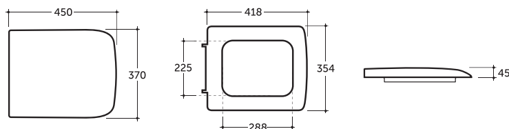
СИДЕНЬЕ С КРЫШКОЙ КВАДРО SLIM (ДЮРОПЛАСТ С МИКРОЛИФТОМ) QUADRO SLIM WC SLIM SEAT WITH COVER (DUROPLAST)
