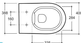
СИДЕНЬЕ С КРЫШКОЙ БЕРГАМО SLIM (ДЮРОПЛАСТ С МИКРОЛИФТОМ) BERGAMO SLIM WC SEAT WITH COVER (DUROPLAST WITH SOFTCLOSE)
