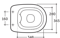
УНИТАЗ БЕЗ ПОЛКИ АЛЬБАНО R НОВА ПЛЮС WC ALBANO R NOVA PLUS WITHOUT SHELF
