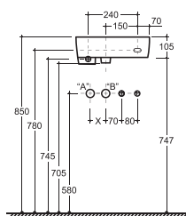
УМЫВАЛЬНИК-РУКОМОЙНИК СКВЭА 36 HAND WASH-BASIN SQUARE 36
